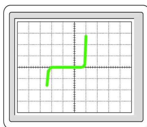
Zener
